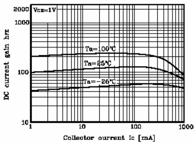
Fig. 5 h_{FE} - I_C
