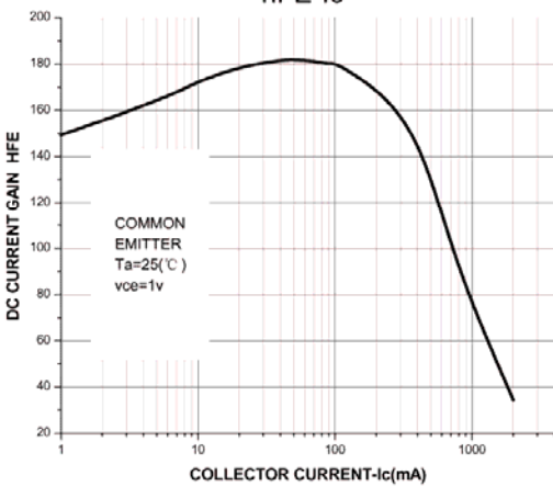
hFE-Ic
